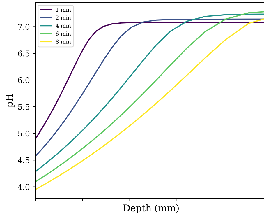
(d) \text{H}_2\text{O}_2
